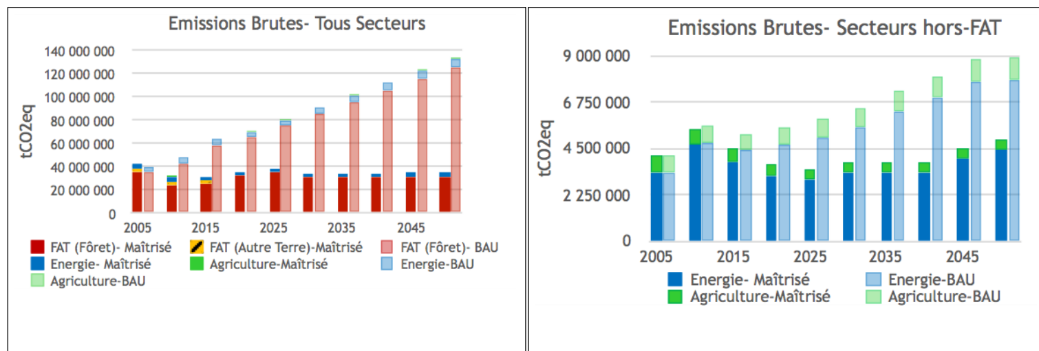
Figure 3. Émissions prévues et scénario de statu quo (BAU) des secteurs FAT, de l'énergie et de l'agriculture. Les données pour 2005-2015 correspondent aux performances réelles (colonnes striées). Les données pour les scénarios sont projetées à partir de 2020 et le scénario de statu quo (BAU) est projeté à partir de 2010 12 .
