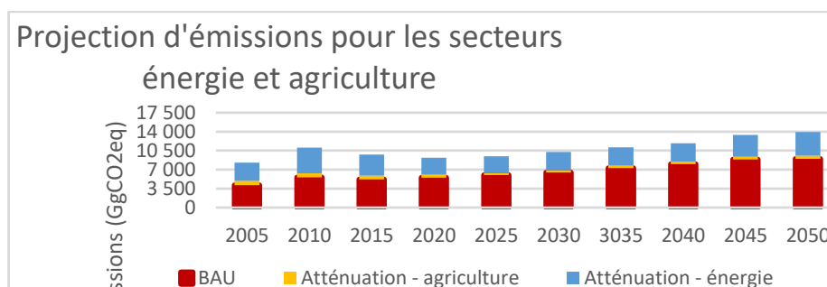
Figure 6 - Émissions des secteurs énergie et agriculture comparé au scénario BAU.
