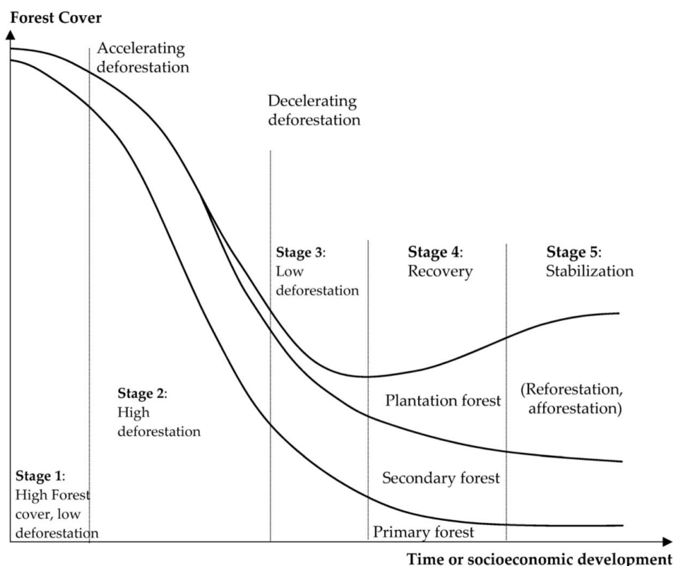
Figure 2. Stades de la courbe de déforestation. 9 Le Gabon est au stade 1.
