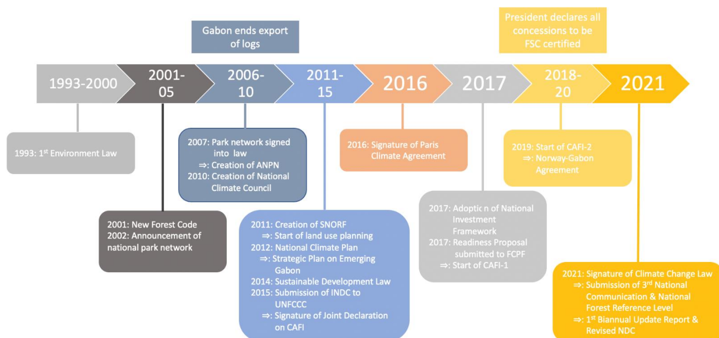
Figure 1. Chronologie des initiatives du Gabon ayant un impact sur les émissions et la séquestration des GES.
