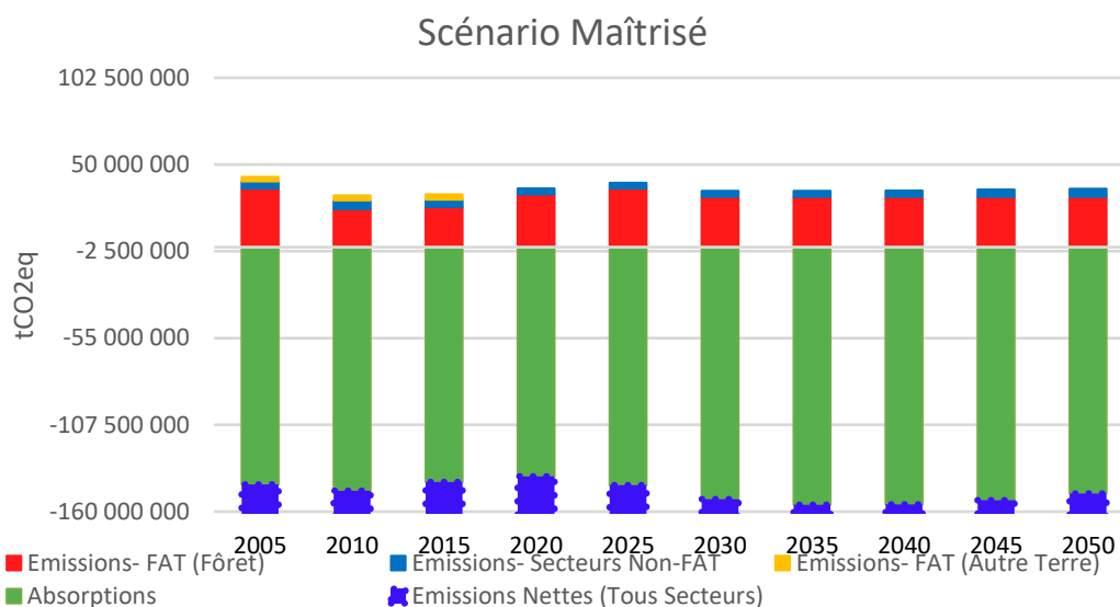
Figure 4. Émissions et séquestrations réelles (colonnes striées) et prévues des secteurs FAT, énergie et agriculture pour la période 2005-2050 et émissions nettes (ou, absorptions nette) 13 .
